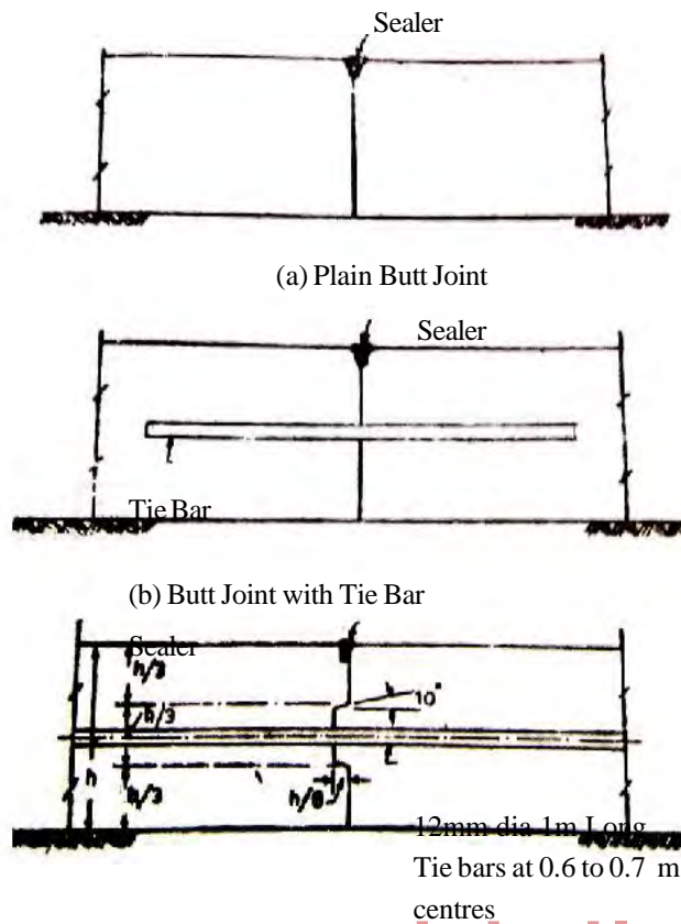
Fig 2.5.6(1) Longitudinal Joints
