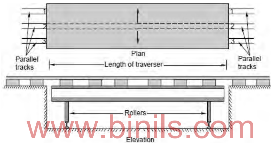
Fig. 4.9 Traverser
