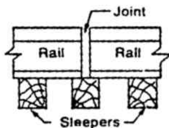
Fig.3.14 (d) Supported joint
