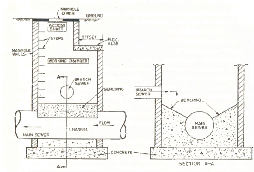
Man hole
